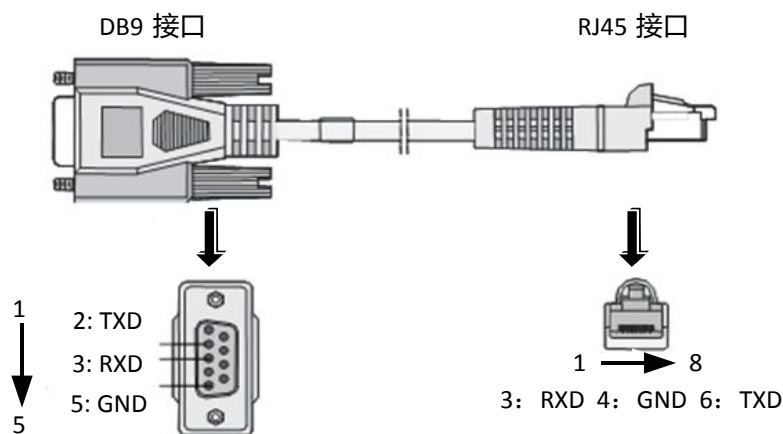
图2-11 RS232 串口线
