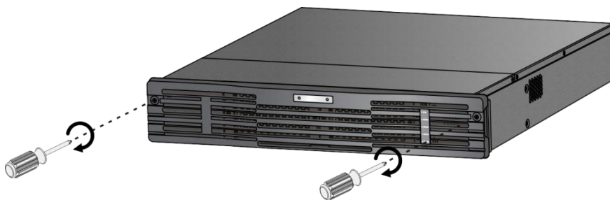
图2-9 安装前面板
