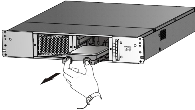
图6-1 拔出硬盘
