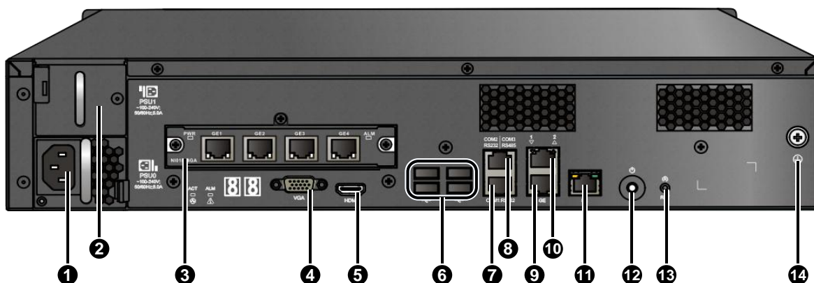
图1-3 后面板接口/按钮
