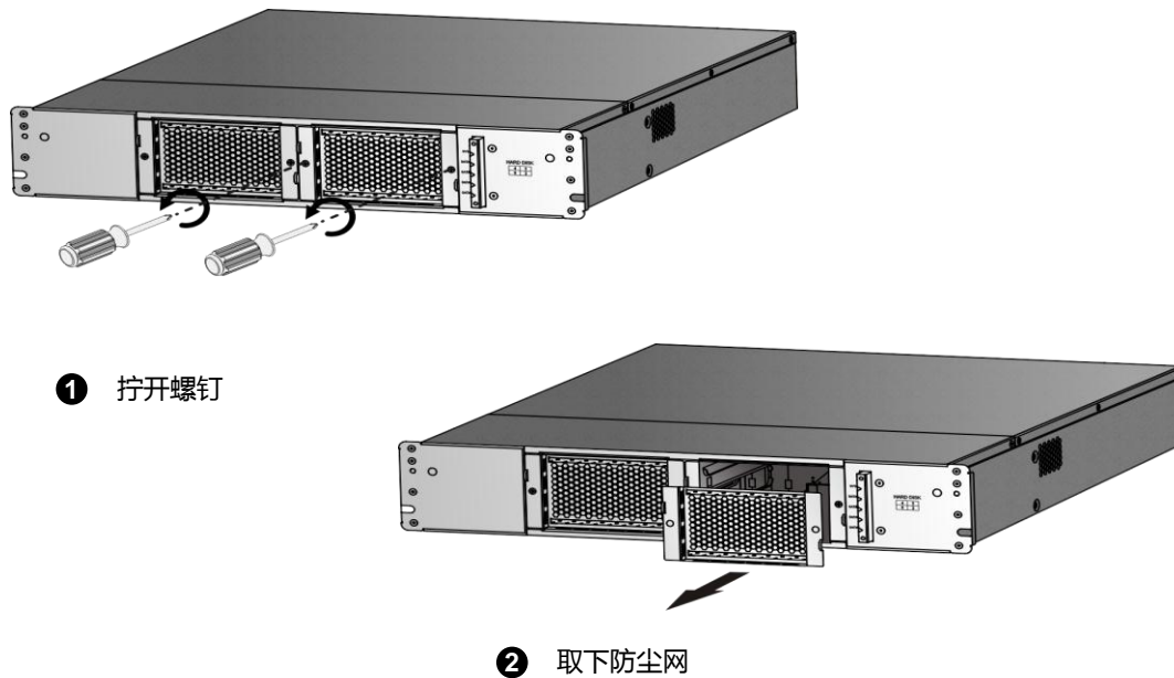
图2-6 拆卸防尘网
